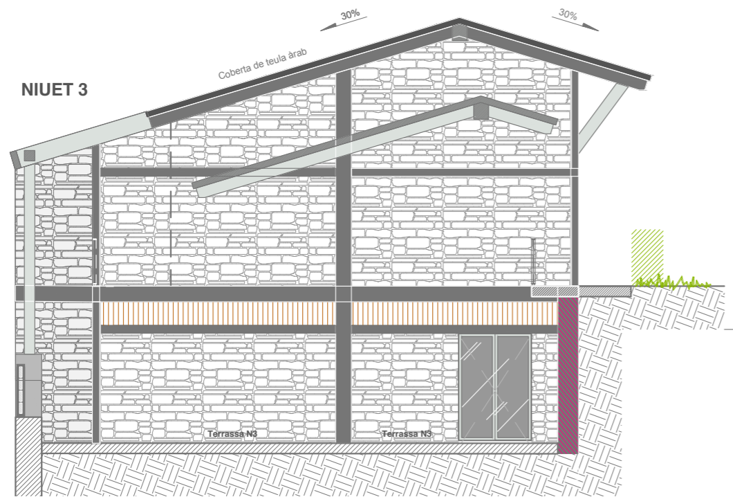
A5 Alçat Lateral Interior NIUET 3
