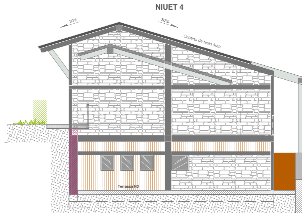
A6 Alçat Lateral Interior NIUET 4
