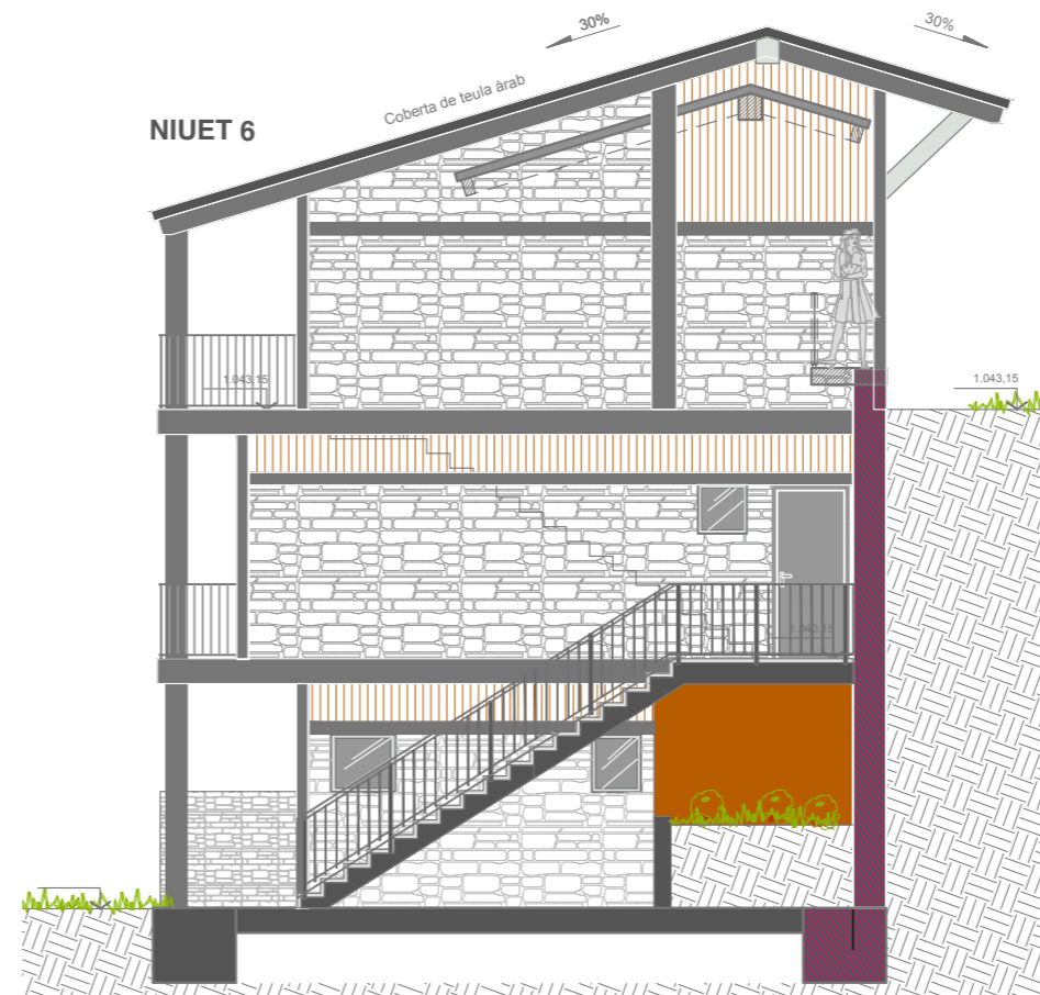
A10 Alçat Lateral NIUETS 5-6-7
