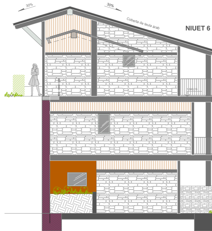
A9 Alçat Lateral NIUETS 5-6-7
