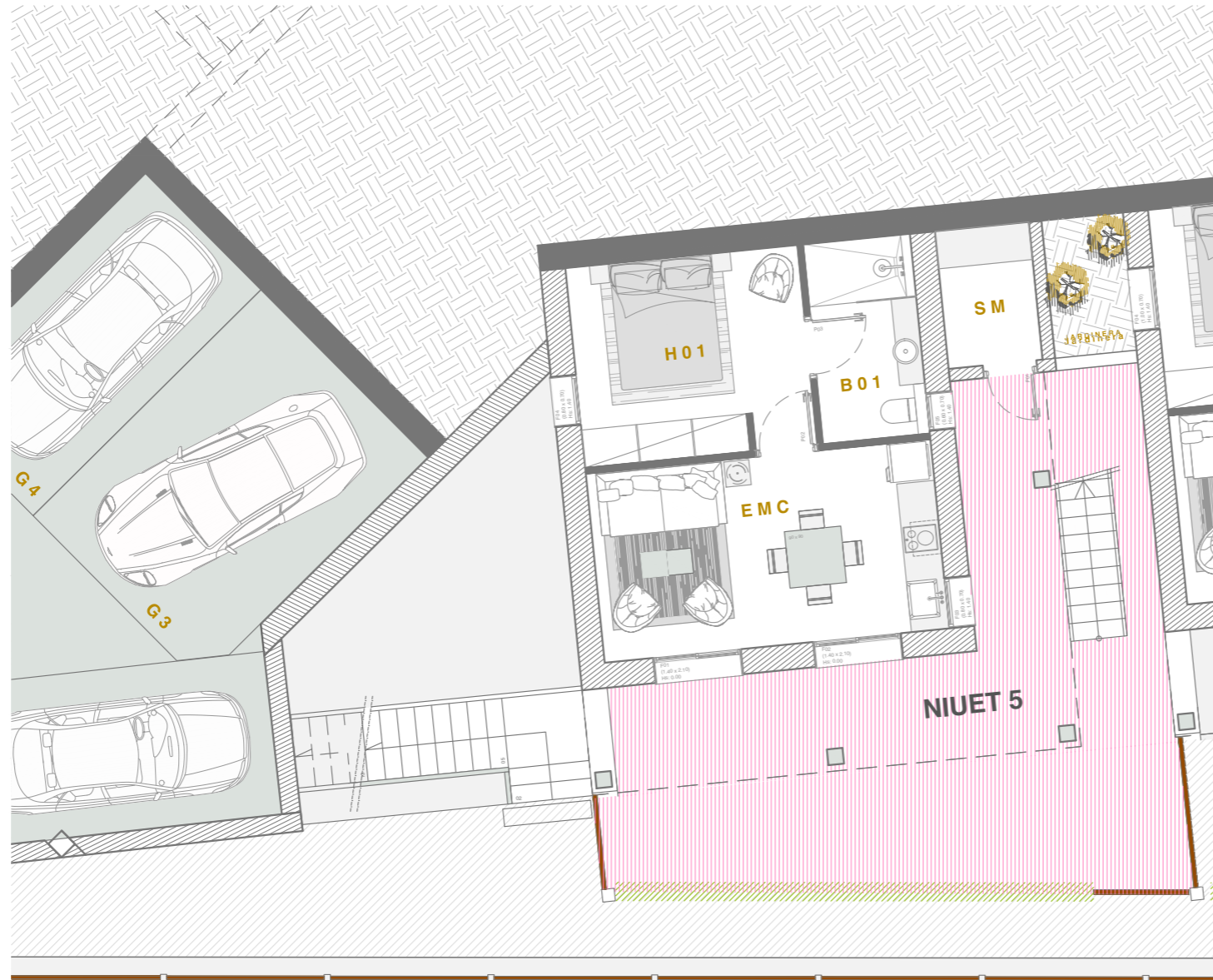
Planta -2
